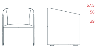
Poltroncina bassa su piedini 1PL6022: L 56 P 57,5 H 67,5
