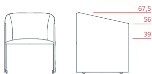
Poltroncina bassa con rotelle 1PL6021: L 56 P 57,5 H 67,5
